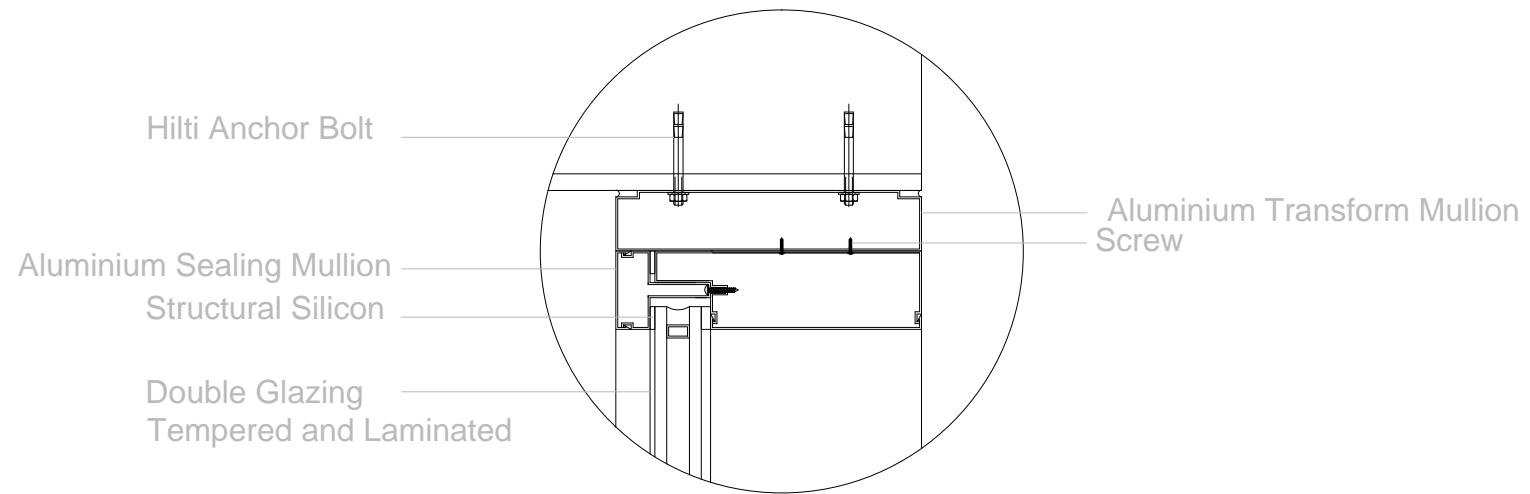
Detail A Scale: 1:5
