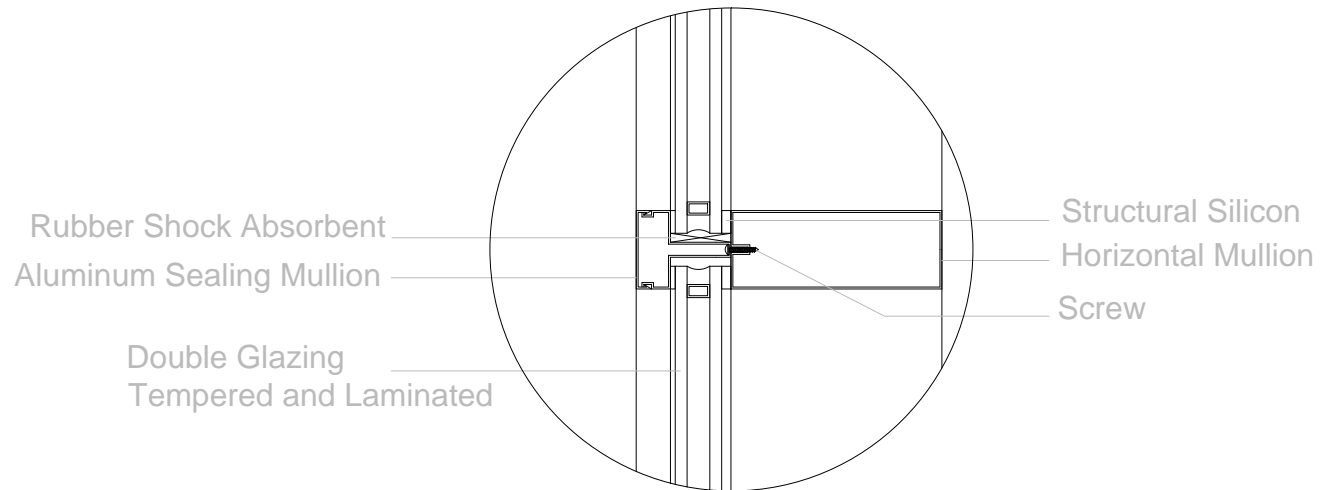
Detail B Scale: 1:5
